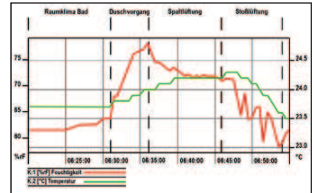
Originalausdruck Datenlogger
